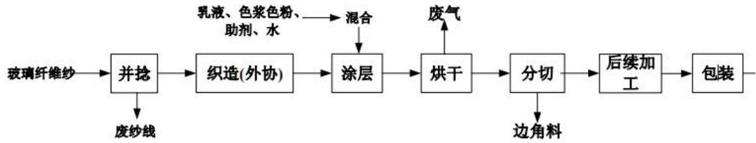
图2 玻纤涂层布生产工艺
