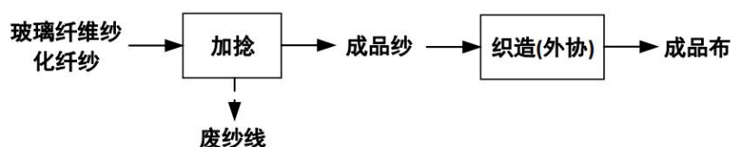
图1 玻璃纤维纱及玻璃纤维布生产工艺
