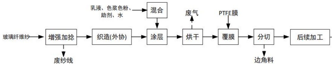
图3 覆膜网格布生产工艺
